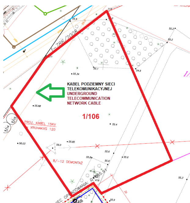
Rys.1. Lokalizacja przebiegu kabla podziemnego sieci telekomunikacyjnej na działce nr 1/106. Fig.1. Location of the underground cable of the telecommunications network on plot no. 1/106.
